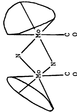
B. Planar-cis ( C_{2v} )
