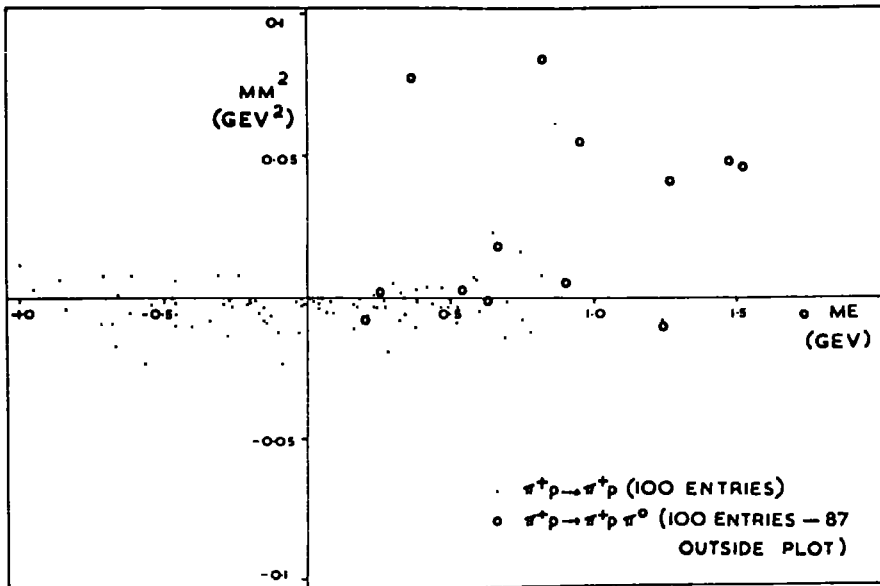
A. 11.5 GEV/c
