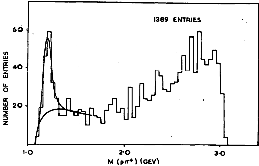
A. M(\rho\pi^+)
