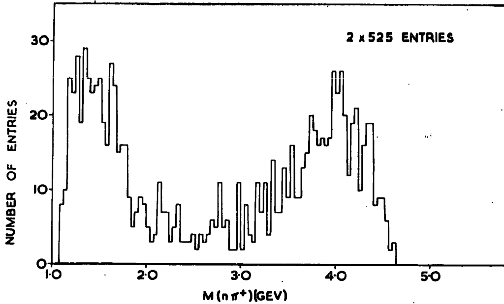
A. M(n\pi^+)
