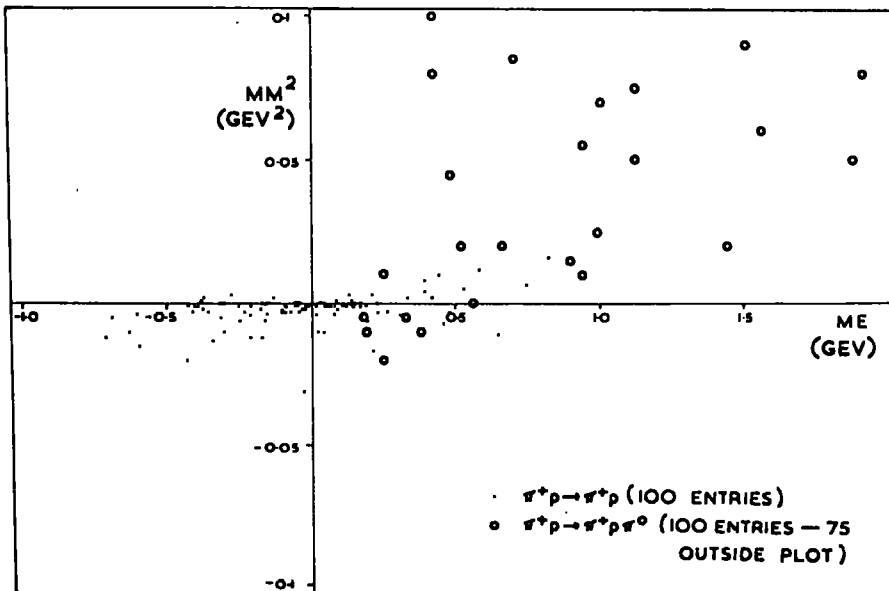
B. 5 GEV/c
