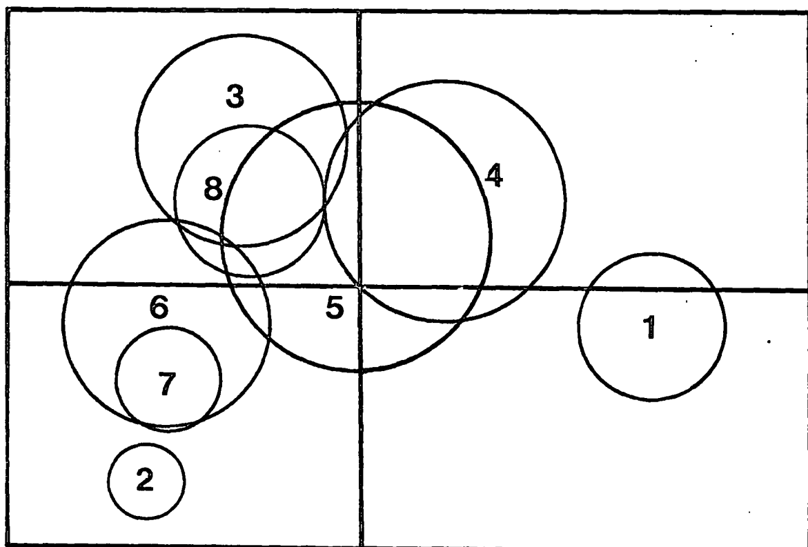
PC 1
