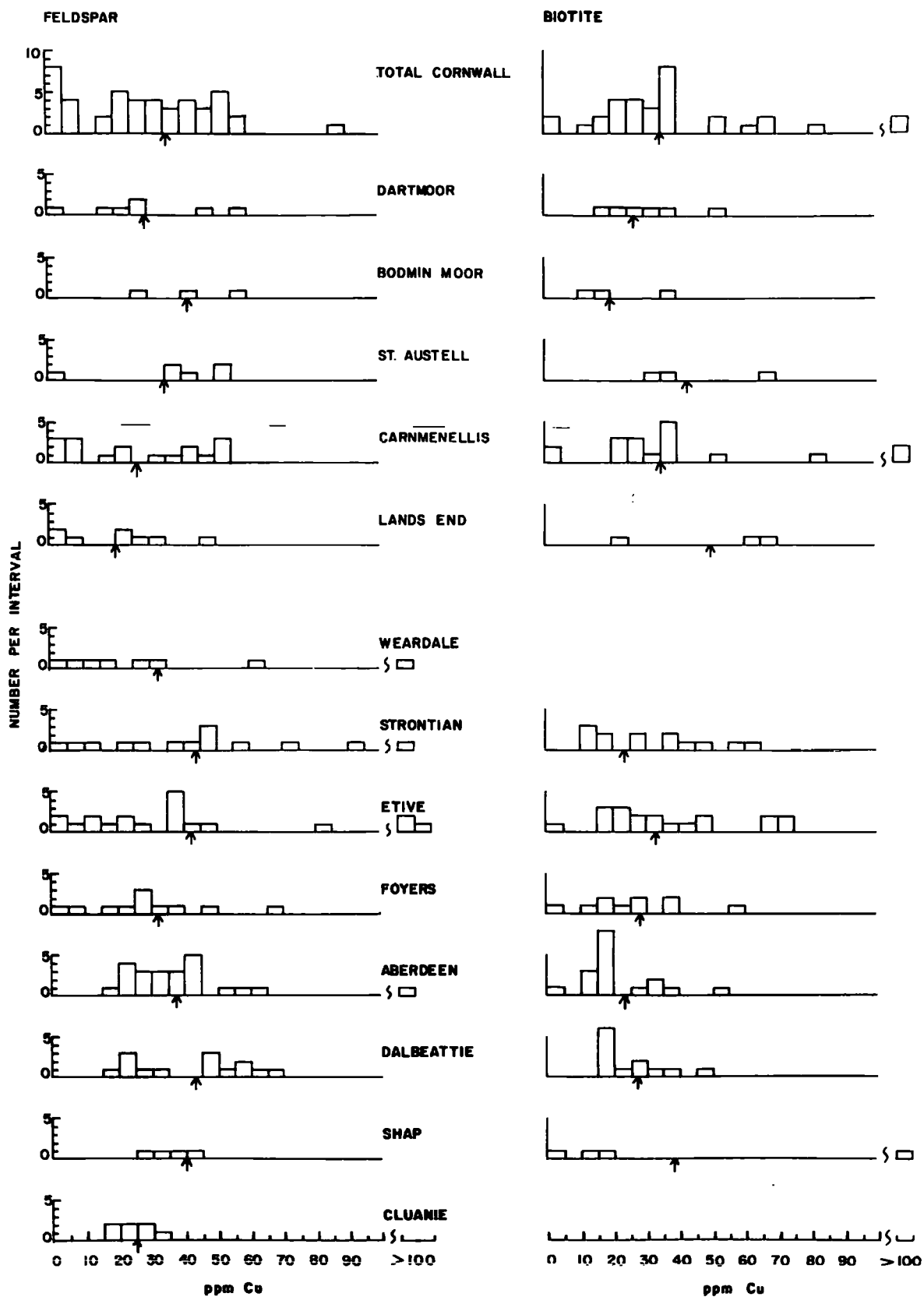
DIAGRAM 17 Cu ANALYSES
