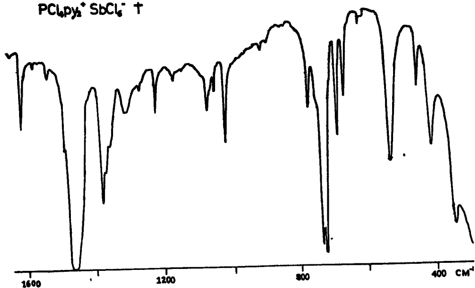
Fig15 Ir spectra 1650-300 cm -1
