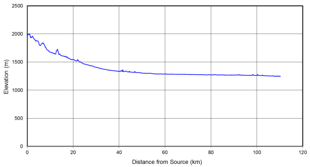
Zamani longitudinal profile
