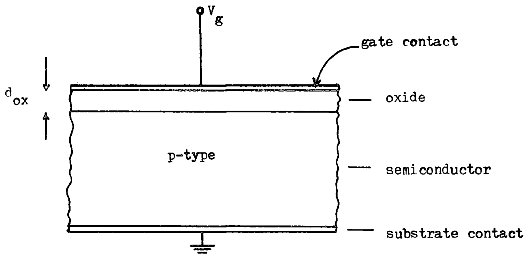
Fig. 2.1 : MOS capacitor structure,
