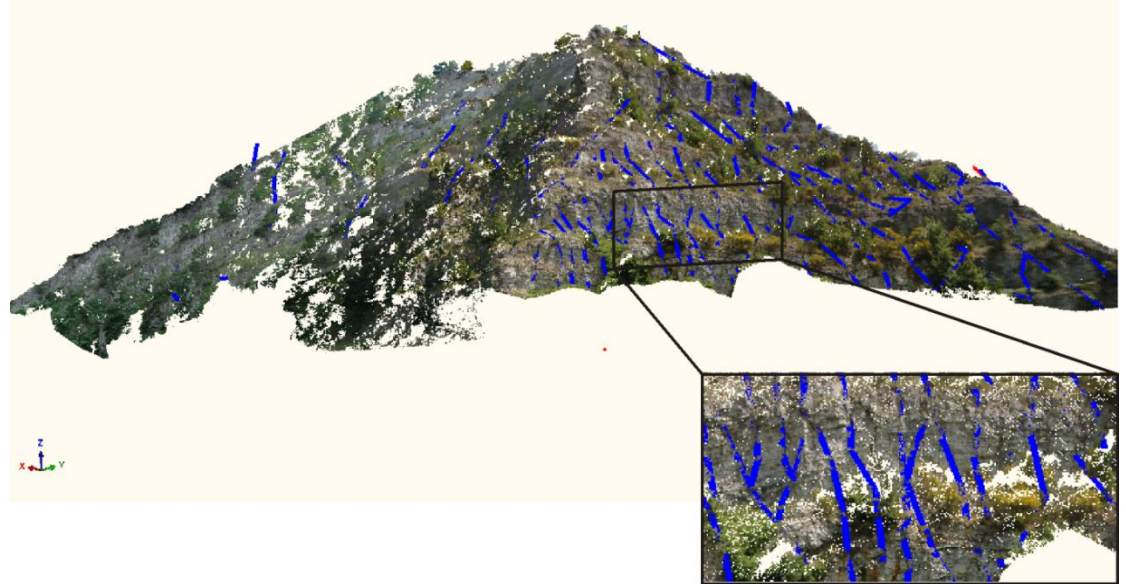
b) Interpreted LiDAR data
