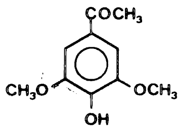
Acetosyringone
