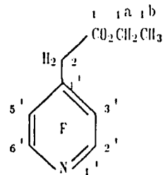
Spectra #25b
