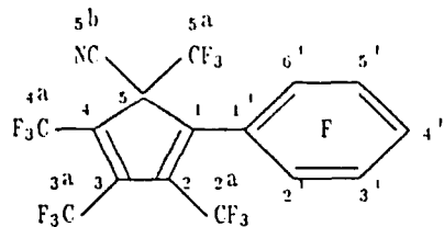
Spectra #63a
