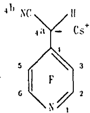
Spectra #25a
