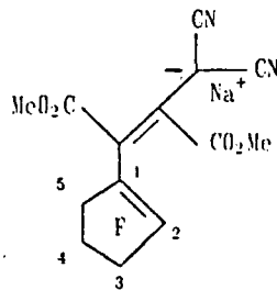
Spectra #63b
