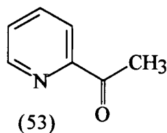
2-acetylpyridine
