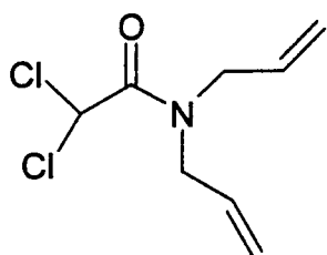
dichlormid
