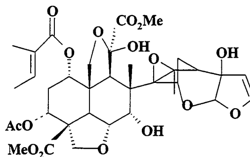
( 9 ) azadirachtin
