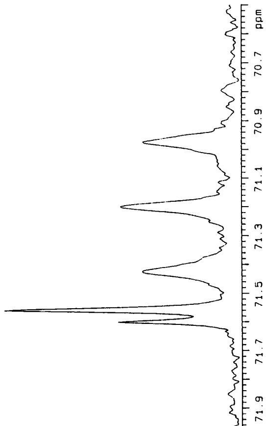
littorine C-2'
