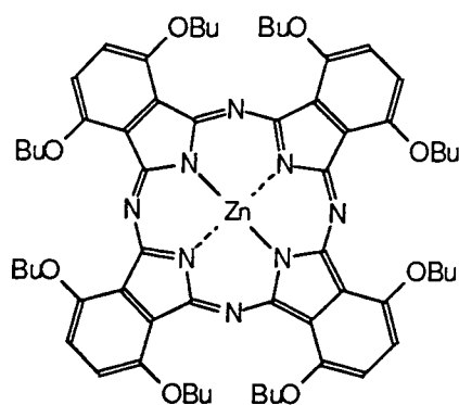
(BuO) 8 ZnPc
