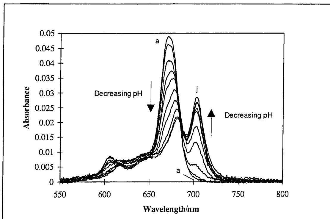
Figure 5.12. Absorbance spectra of \text{ZnPcS}_2 in buffers ranging from pH 7 to 1. \text{pH}=\text{a) } 7.06 \text{b) } 5.8 \text{c) } 5.3 \text{d) } 4.56 \text{e) } 4.17 \text{f) } 3.48 \text{g) } 3.38 \text{h) } 2.5 \text{i) } 2.1 \text{j) } 1.06 .
