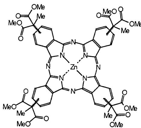
ZnPc(CMe(CO 2 Me) 2 ) 4
