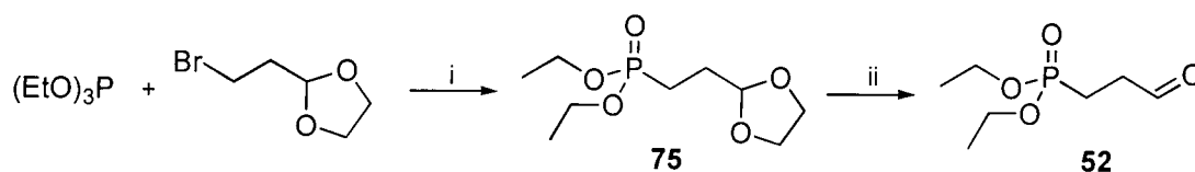
Scheme 23 i. 4 h, 145 °C, 1 h, 165 °C, 85 %; ii. 0.1 M HCl (aq) , 3 h, reflux, 98 %.
