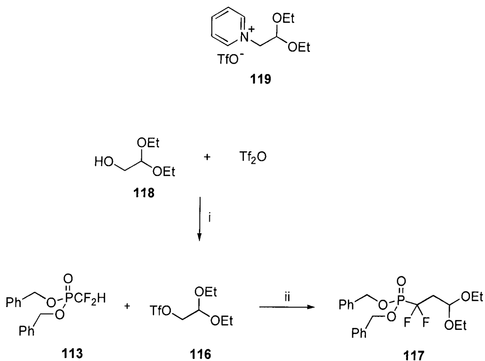
Scheme 52 i. DTBP, CH 2 Cl 2 , 25 min, -20 °C, ~ 65 %; ii. LDA, THF / HMPA, 2 h, -78 °C, < 10 %.
