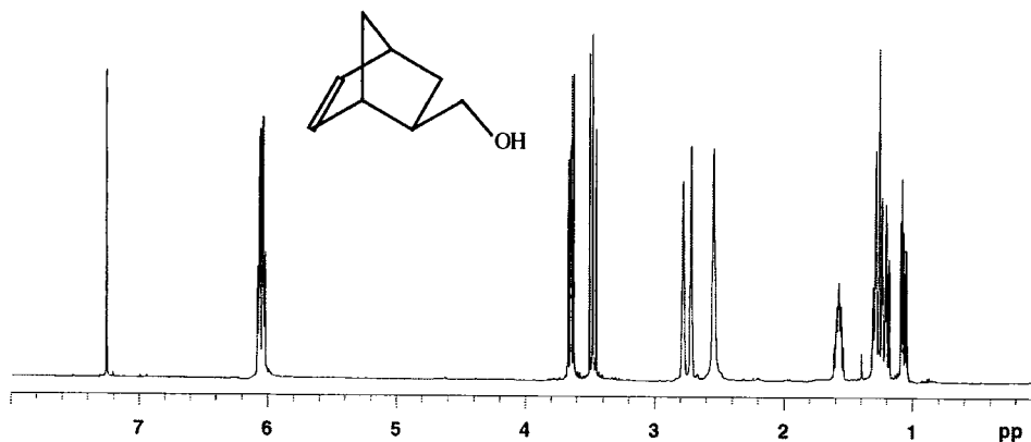
1 H-NMR spectrum (CDCl 3 , 400MHz).
