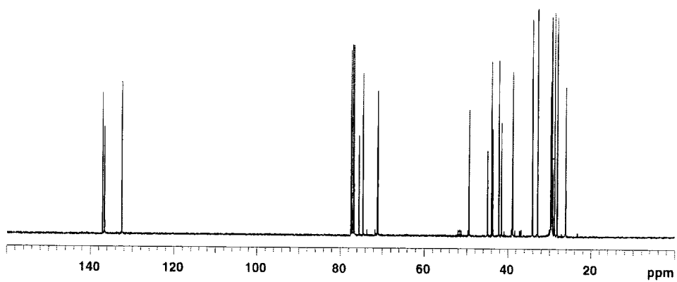
13 C-NMR spectrum (CDCl 3 , 100MHz).
