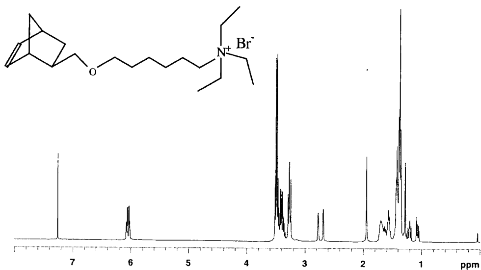
1 H-NMR spectrum (CDCl 3 , 400MHz).
