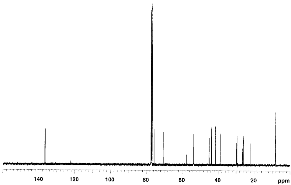
13 C-NMR spectrum (CDCl 3 , 100MHz).
