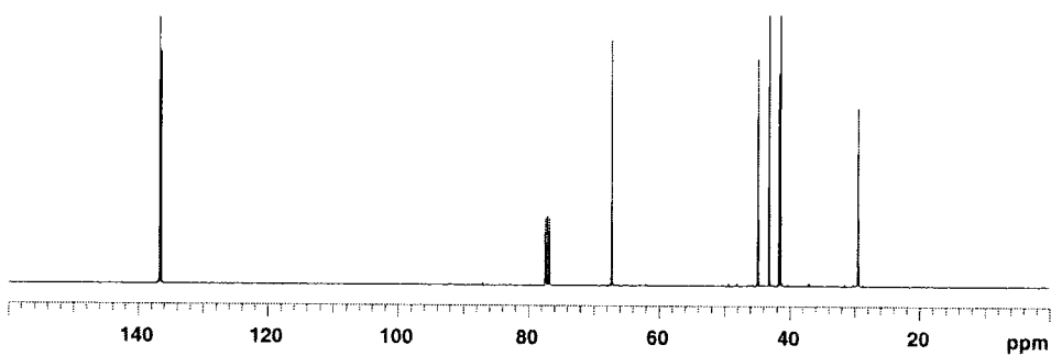
13 C-NMR spectrum (CDCl 3 , 100 MHz).
