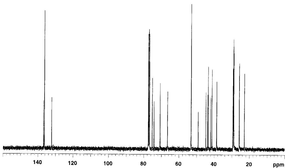
13 C-NMR spectrum (CDCl 3 , 100MHz).
