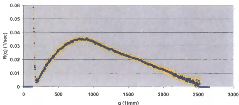
EB25X5 160°C R(q) vs q
