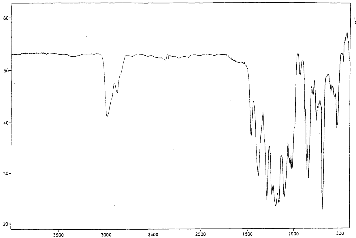
No. 29 tris(2,2,3,4,4,4-hexafluoro-1-methylbutyl)amine (106)
