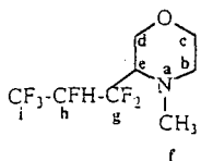
No. 36 4-(2,2,3,4,4,4-hexafluorobutyl)morpholine (113)
