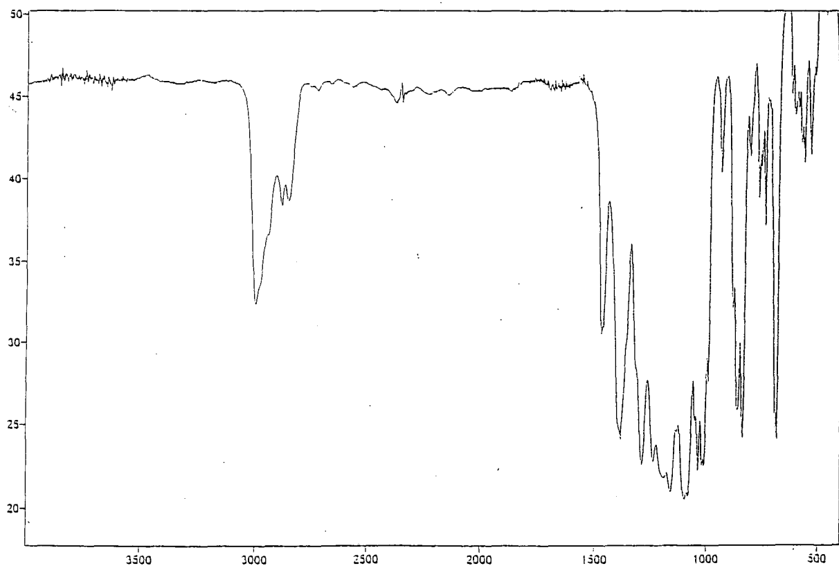
No. 27 diethyl(2,2,3,4,4,4-hexafluoro-1-methylbutyl)amine (104)
