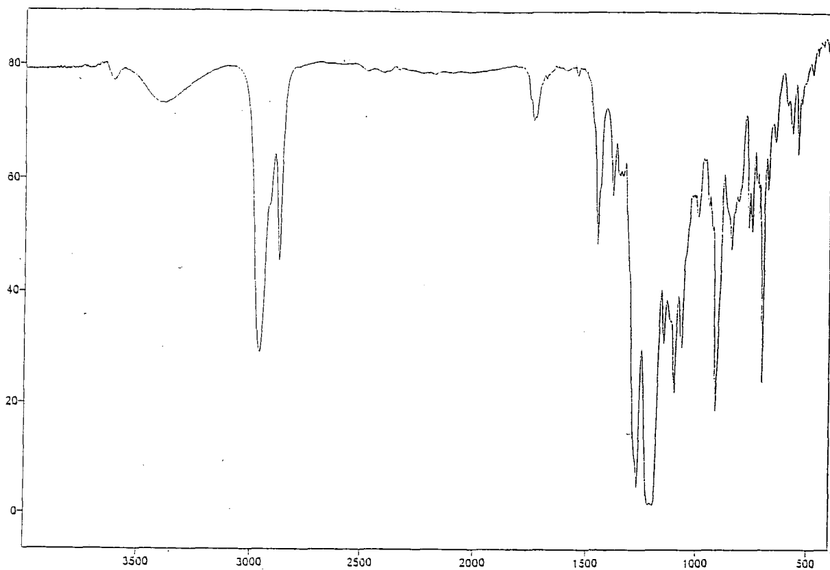
No. 27 diethyl(2,2,3,4,4,4-hexafluoro-1-methylbutyl)amine (104)
