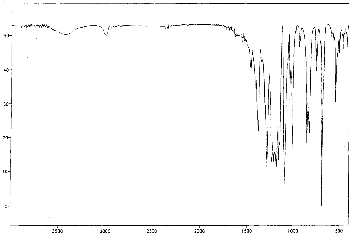
No. 29 tris(2,2,3,4,4,4-hexafluoro-1-methylbutyl)amine (106)
