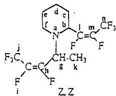
No. 42 1-((Z,Z)-2,3,4,4,4-pentafluoro-1-methylbut-2-enyl)-2-((1Z)-1,2,3,3,3-pentafluoroprop-1-enyl)piperidine (119)
