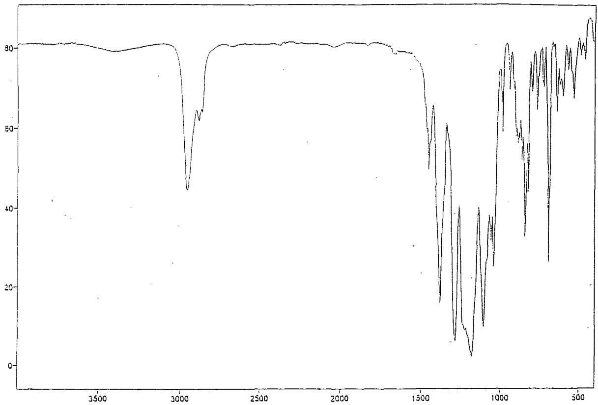
No. 35 1-(2,2,3,4,4,4-hexafluoro-1-methylbutyl)-2-(1,1,2,3,3,3-hexafluoropropyl) piperidine (112)
