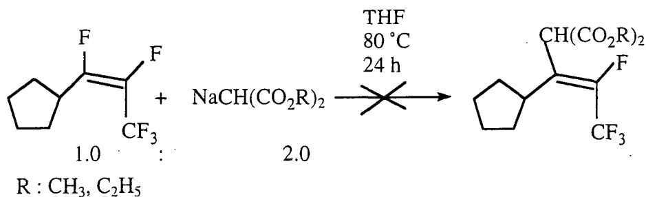
Scheme 158
