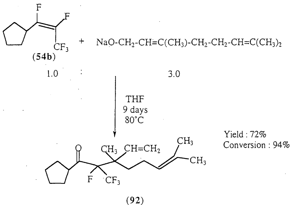
Scheme 145
