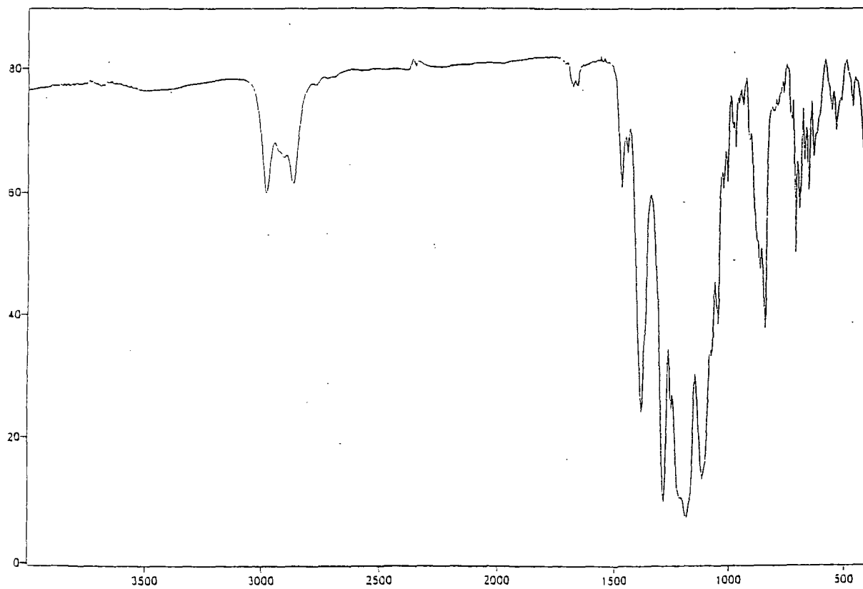
No. 37 4-(2,2,3,4,4,4-hexafluorobutyl)-3-(1,1,2,3,3,3-hexafluoropropyl)morpholine (114)
