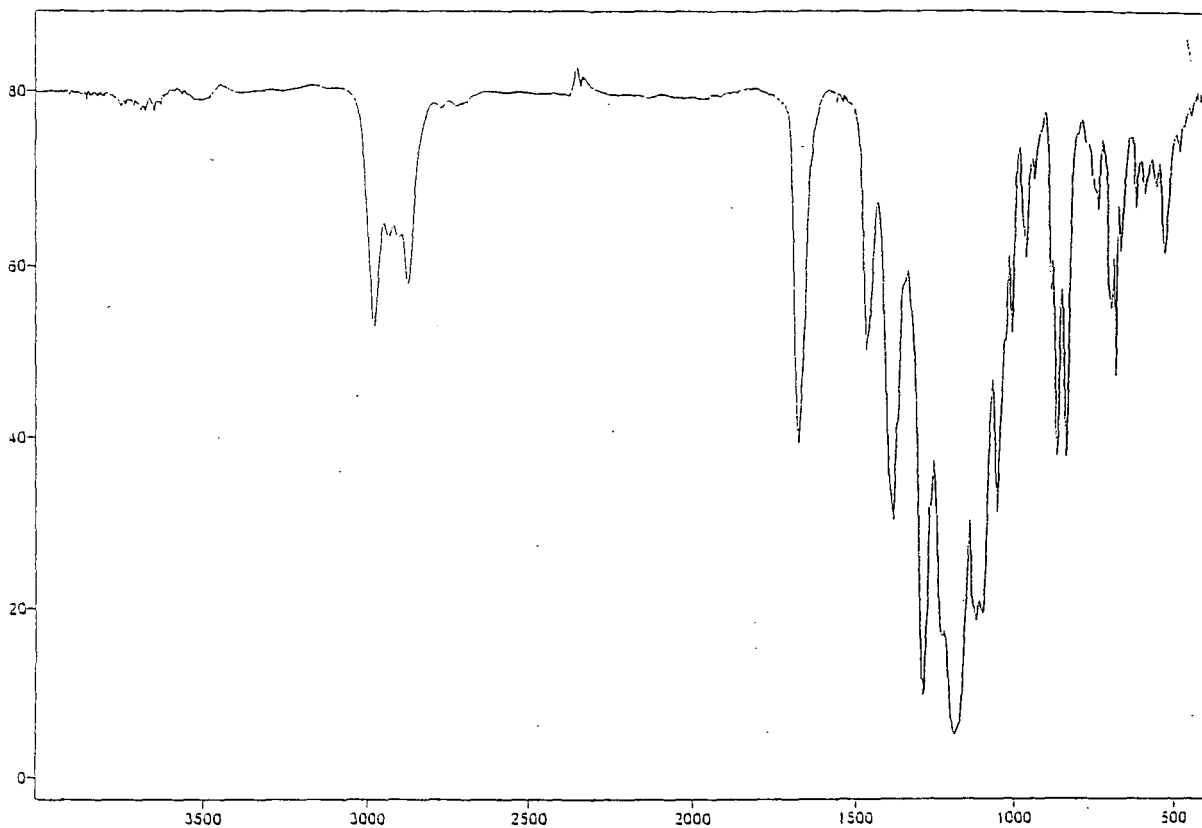
No. 39 4-(2,2,3,4,4,4-hexafluoro-1-methylbutyl)-3-(1,1,2,3,3,3-hexafluoropropyl) morpholine (116)
