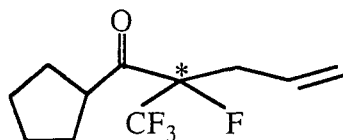
Scheme 135
