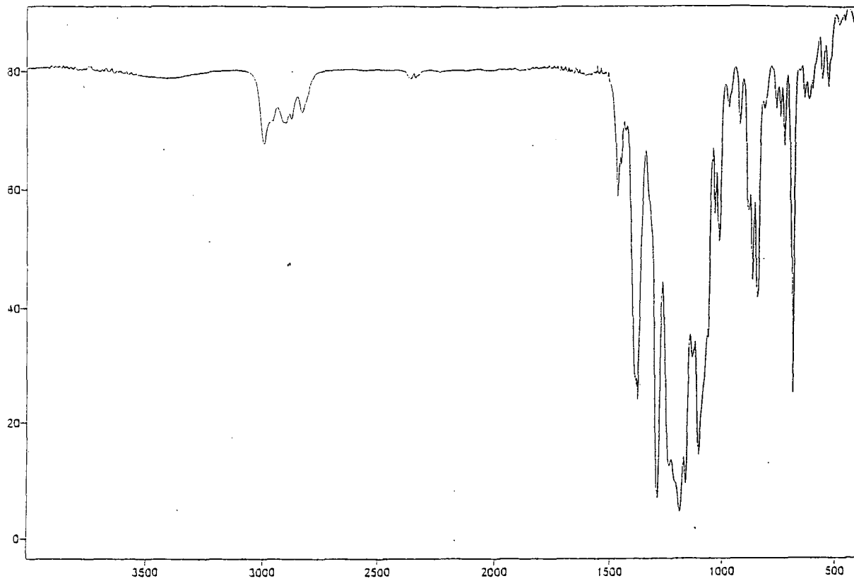
No. 31 bis(methylethyl)(2,2,3,4,4,4-hexafluoro-1-methylbutyl)amine (108)
