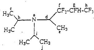
No. 31 bis(methylethyl)(2,2,3,4,4,4-hexafluoro-1-methylbutyl)amine (108) Minor Diastereoisomers
