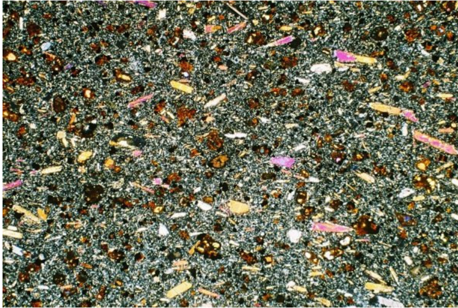
Plate 10: G069 (Wadi al-Khaymat), nephelinite in XPL
