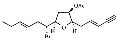
(+)- trans -kumausyne
