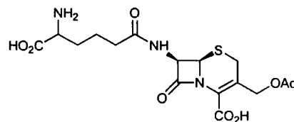
5 Cephalosporin C
