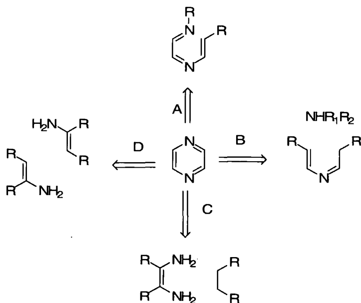
Scheme 1.4
