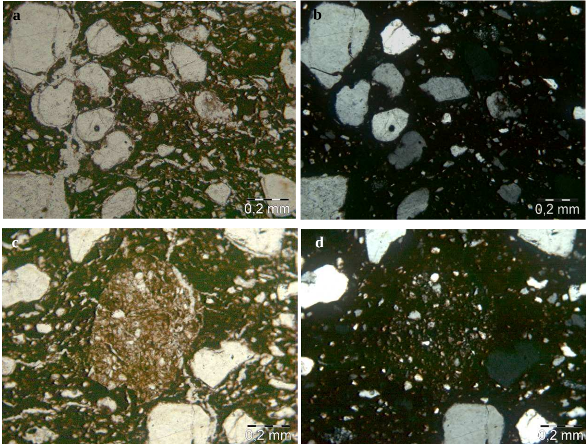
Figures 78 : Bdx11983 : Images au microscope polarisant, lumière polarisée non analysée (a & c) et polarisée analysée (b & d) x100 : abondance de très grosses inclusions dans une pâte fine. On note un réseau poreux important.
