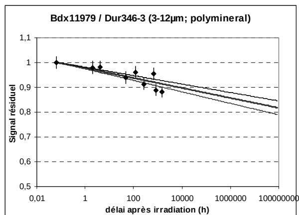
Figure 81 : Bdx 11979/Dur346-3: Étude de la stabilité des signaux de TL : existence d'un fading , qui n'atteint pas de niveau stable après 2 mois de délai. La courbe ajustée aux points expérimentaux correspond à une loi déduite du modèle de recombinaison par effet tunnel (de type logarithmique). L'ajustement selon un modèle de décroissance logarithmique caractéristique des pertes par effet tunnel des feldspaths convient.
