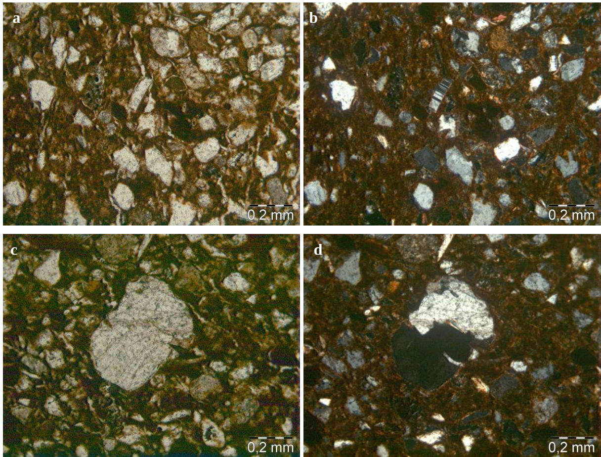
Figures 89 : Bdx11984 : Microscope polarisant : lumière polarisée non analysée (a, c) et polarisée analysée (b, d) x100 : abondance d'inclusions comprises entre 80 et 200 \mu m, réparties de manière homogène. a et b montrent la présence de feldspaths plagioclases et c et d la présence ponctuelle de grains de diamètre supérieur à 0,5mm et la présence de grains de fer inclus dans ces grains.
