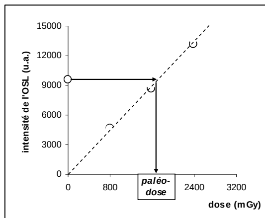
Figure 28: Détermination de la dose d'irradiation archéologique à partir d'une série d'expériences obtenues par l'ajout de doses sur aliquote préalablement vidée de son OSL naturelle (par éclairage). La valeur de la paléodose est déterminée par interpolation de l'intensité de l'OSL naturelle sur la loi d'acquisition (intensité de la luminescence en fonction de la dose d'irradiation bêta administrée).
