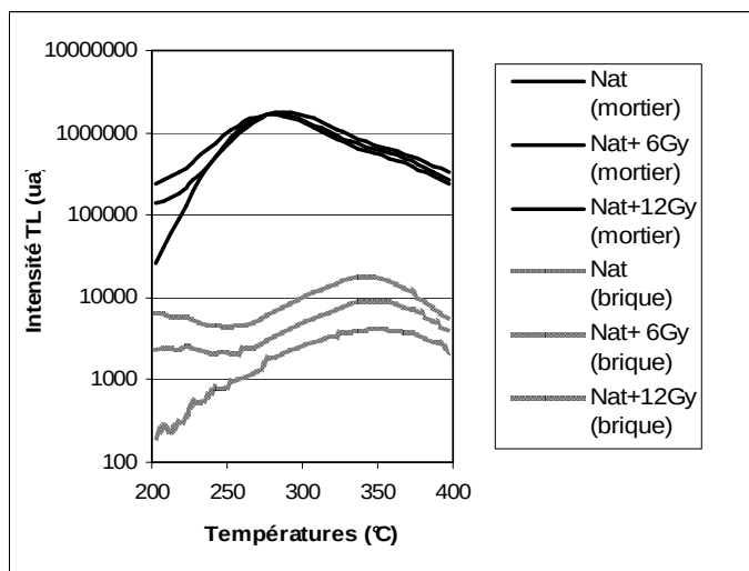
Figure 64 : Comparaison entre les courbes TL du mortier (en noir) et celles des briques (en gris) (échelle logarithmique).
