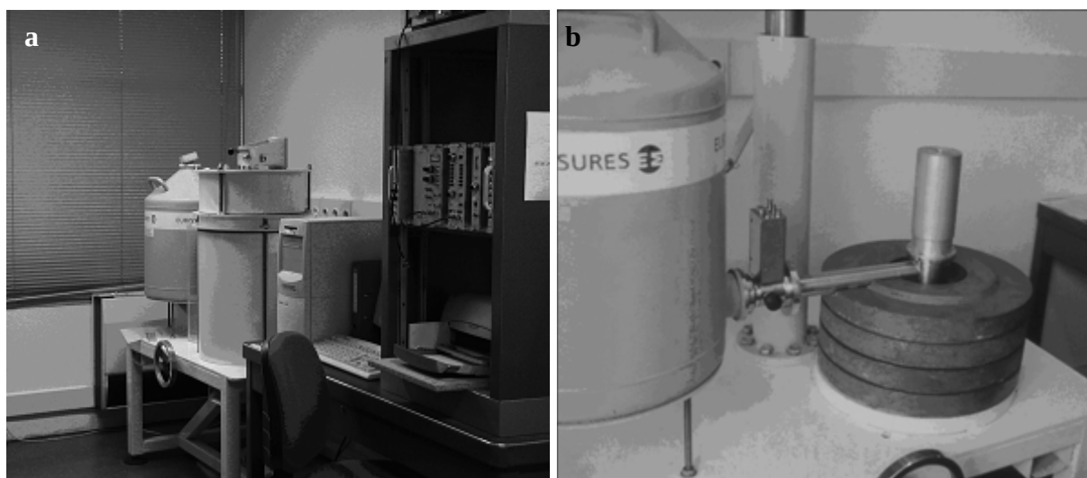
Figures 31 a & b: appareillage de spectrométrie gamma à bas bruit de fond utilisé au laboratoire de Bordeaux (de type EGPC 200 P 17, Eurisys Mesures). Le dispositif s'organise autour d'un détecteur germanium puits, refroidi à l'azote liquide. Le détecteur est entouré d'une couronne de plaques de plomb de faible activité, destinées à absorber le rayonnement \gamma provenant de l'environnement du détecteur (photos IRAMAT-CRP2A).
