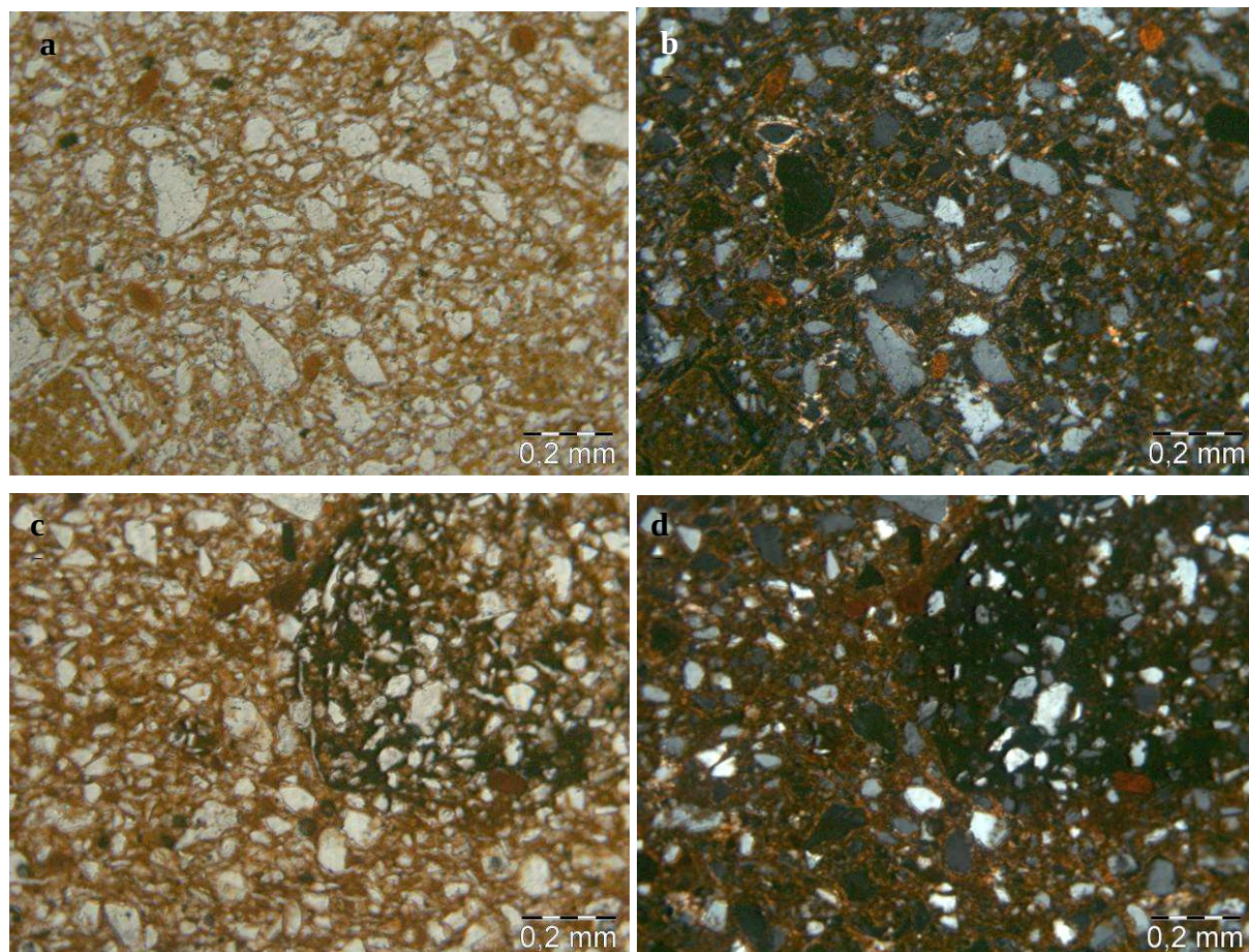
Figures 104 a, b, c & d : Observation (x100) en lumière polarisée non analysée (a, c) et polarisée analysée (b, d) de la lame mince de l'échantillon Bdx11989. On observe que la pâte est relativement homogène quant à la nature, à la fréquence, à la taille et à la proportion des inclusions qu'elle contient : l'échantillon présente une texture très chargée en petites inclusions.
