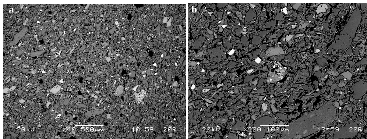
Figures 53 : Bdx9457 : images MEB en mode électrons rétrodiffusés; grossissement x40 (a) et x200 (b) inclusions comprises entre 80 et 200 μm en quantité insuffisante pour répondre au besoin de la préparation de quartz des échantillons en vue de leur datation par la méthode des grandes inclusions.
