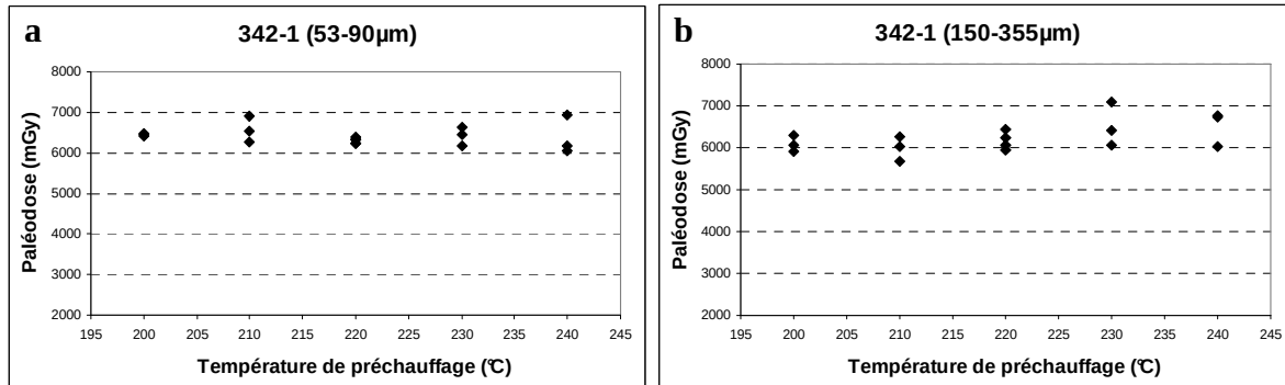
Figures 143 a & b : plateaux de préchauffage de l'échantillon 342-1 pour les granulométries 53-90 μm (a) et 150-355 μm (b). Le préchauffage est maintenu pendant 10s, à une température comprise entre 200 et 240 °C.
