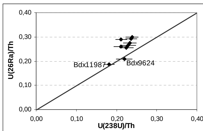
Figures 108: Etude du déséquilibre des séries de l'uranium par l'analyse du rapport des concentrations U(^{238}\text{U})/\text{Th} et U(^{226}\text{Ra})/\text{Th} .
