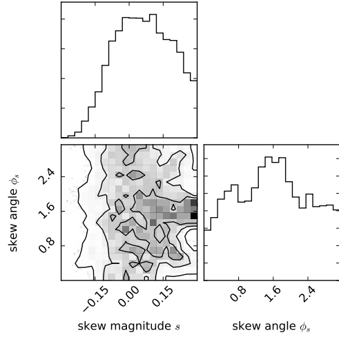
(g) Galaxy N4
