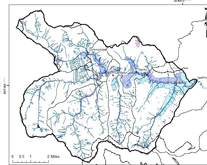
Map 3.5.6. BGS – Superficial Drift Geology
