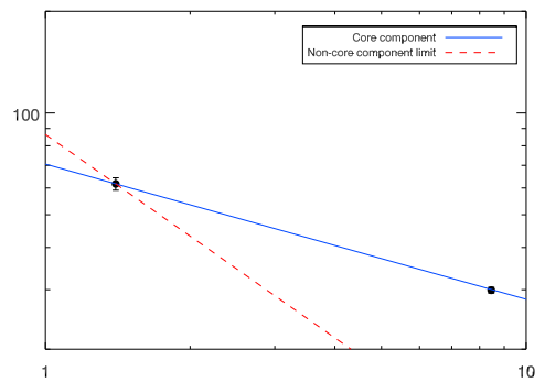
RXJ1504.1-0248
