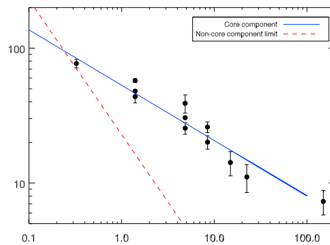
RXJ1715.3+5725/NGC6338
