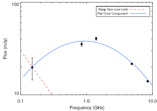
RXJ1304.3-3031
