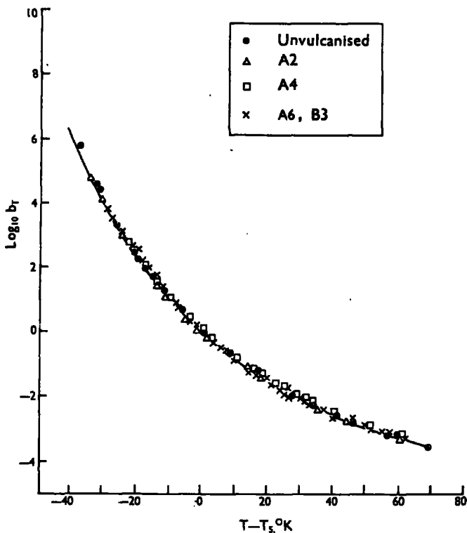
FIG. 13. \text{Log } b_T values.
