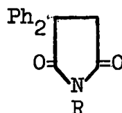
(XV)
